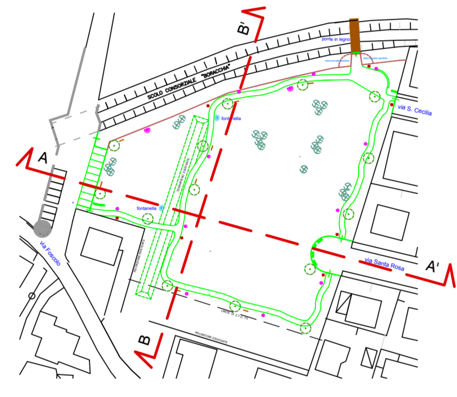
Planimetria 1:1000
